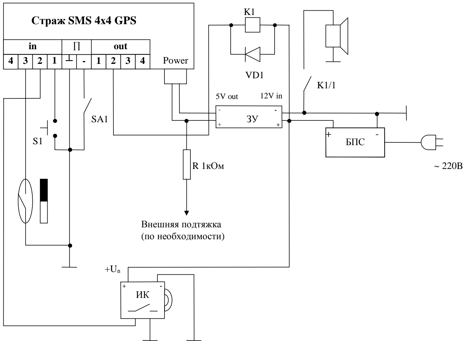
Пример подключения системы «Страж SMS 4x4 GPS» в качестве системы охраны дома
