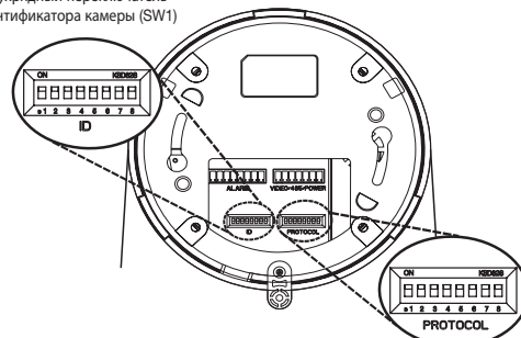
Двухрядный переключатель протокола связи (SW2)
