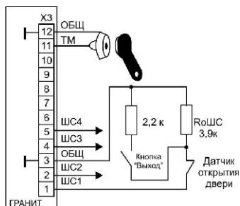
Рис. 7 Подключение цепей управления доступом
